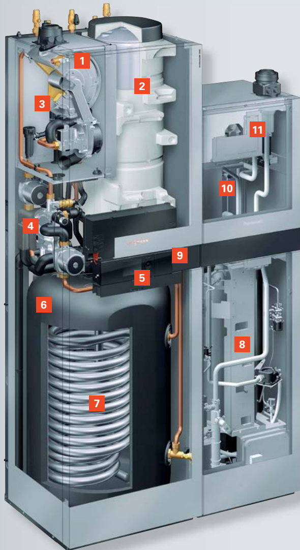
Brennstoffzellen-Heizgerät Vitotalor 300-P
